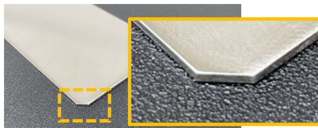
材質：SUS304 板厚：2.0mm
