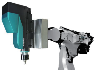
4 ロボットマシニングユニット SDR
